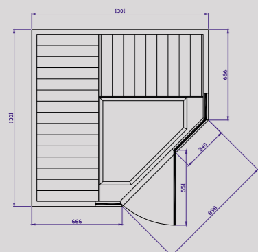
TYLÖSAND T-870 Size: D 1 301 x W 1 301 mm Power: 1600 W
